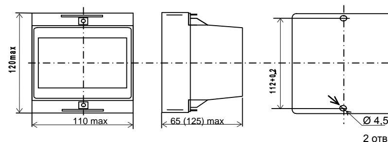
Габаритные и установочные размеры ИП E854M/x, E855M/x
